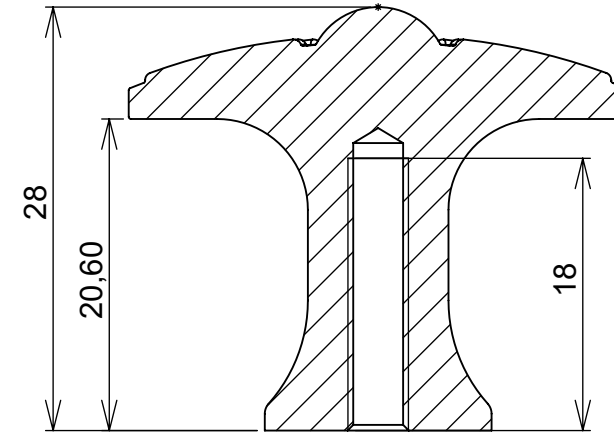
SEÇÃO F-F ESCALA 2 : 1
